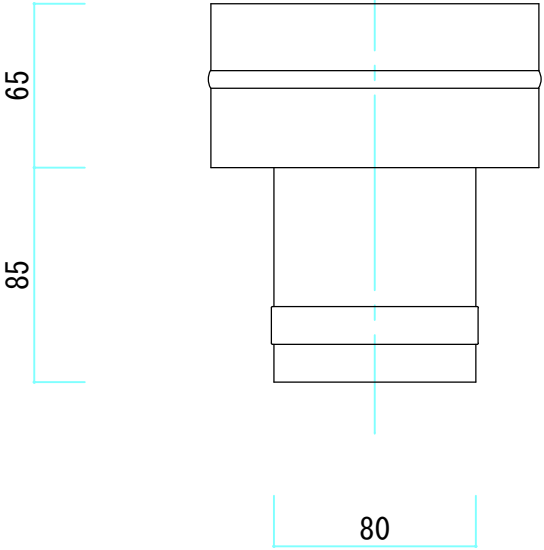
異径ソケット X型
