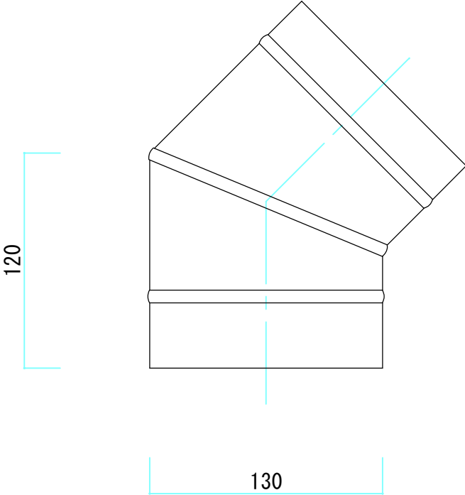
45° エルボ
