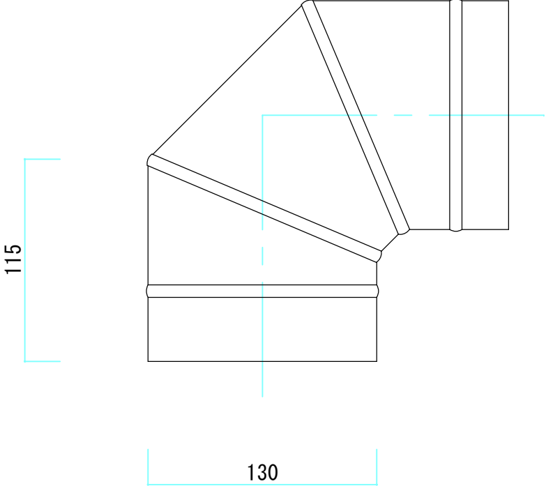
90° エルボ
