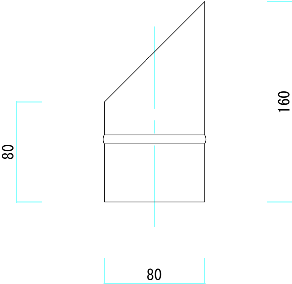
エンドターミナル
