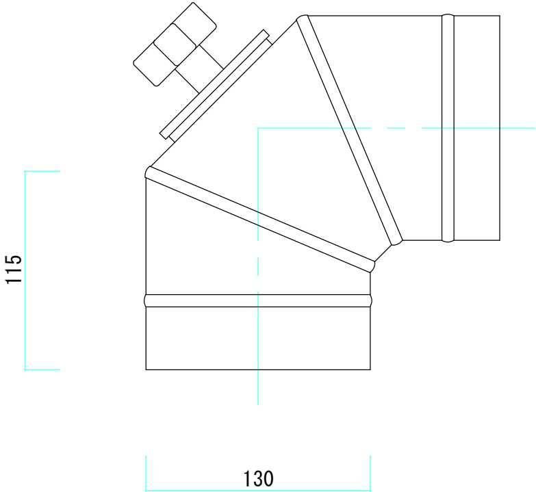
掃除口付エルボ
