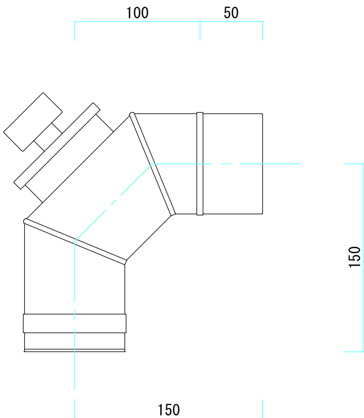
φ80 掃除口付90° エルボ ブラック（ステンレス T=0.5）
