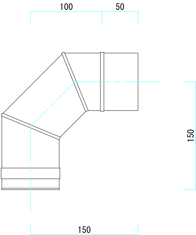
φ80 90° エルボ ブラック（ステンレス T=0.5）
