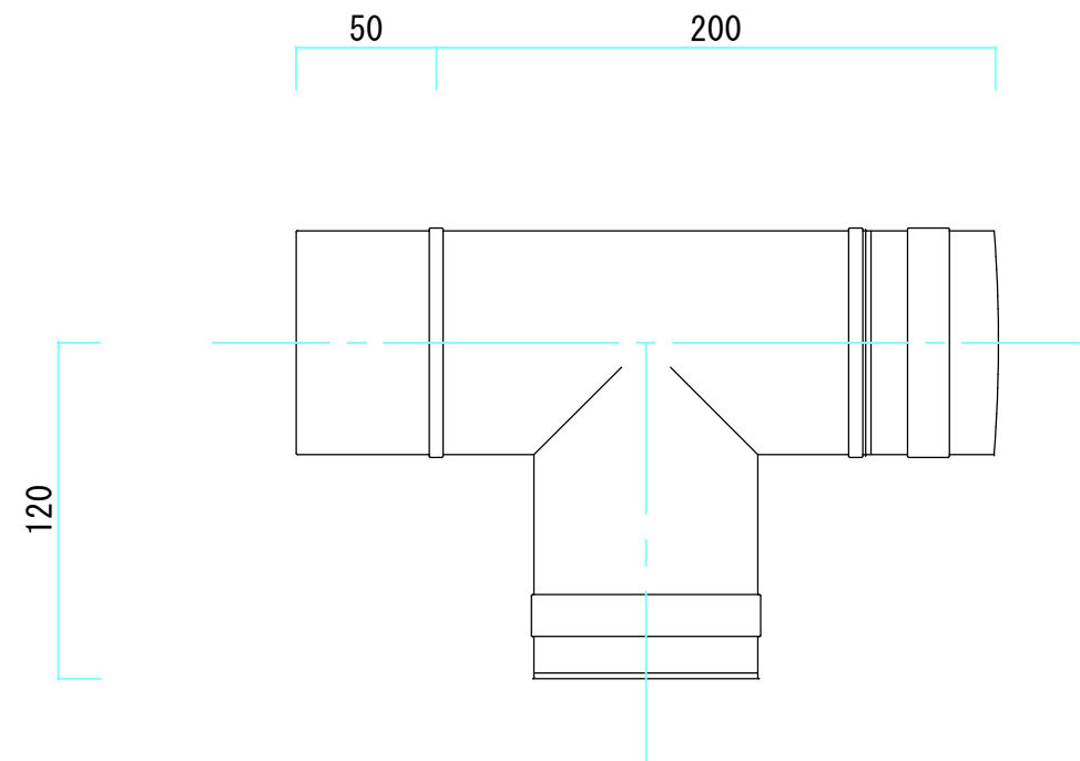
φ80 T字管 灰取フタ付 ブラック（ステンレス T=0.5）
